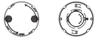
(1) Forgassa el az intelligens kulcs hátlapját és távolítsa el. (2) Vegye ki és cserélje le 1x CR2450 akkumulátóra.
